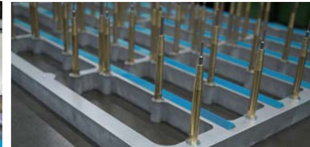
Marco inferior de pines.
